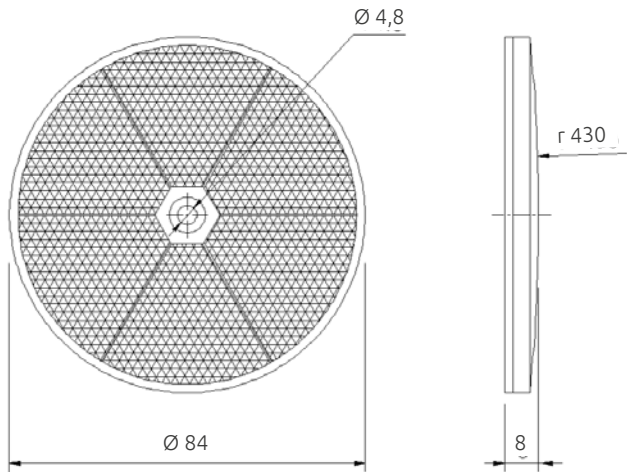
Retro-reflector CD8
